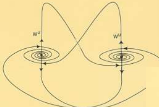
(b) Heteroclinic
